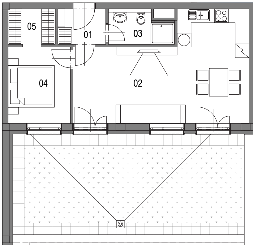
SCHÉMA PODLAŽÍ
